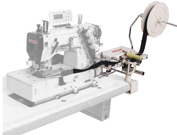
KL-GFS-1 侧送型送带机 Side Tape Feeder
