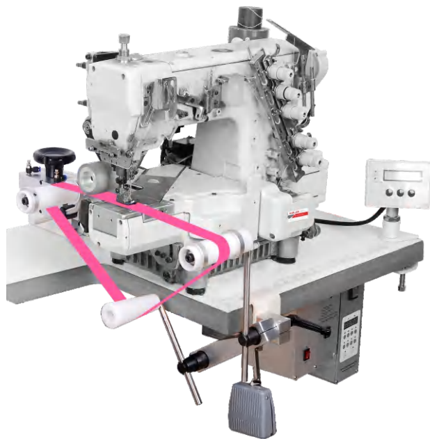
KL-600-01DA/1302 气动裤头滚轮辅助器 Pneumatic Roller Tension Device
